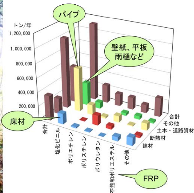
土木建築資材の樹脂別・用途別需要量
