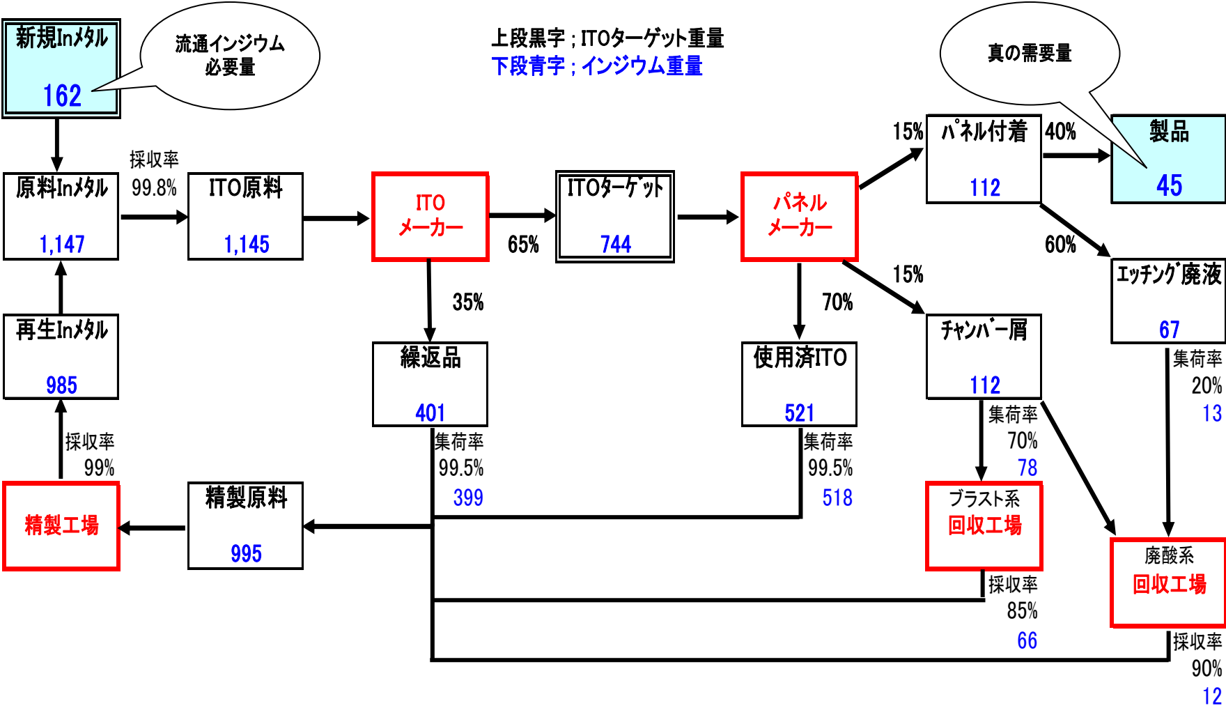
ITOターゲット製造フローとInメタルバランス(マーケット静止時)
